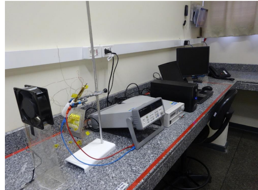
Desempenho térmico de tubos de calor
