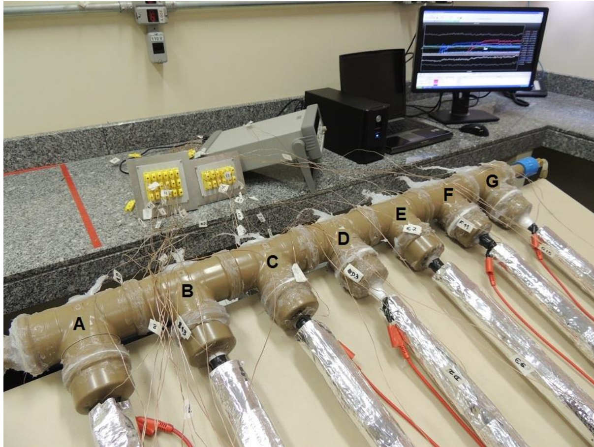
Protótipo de um coletor solar assistido por termossifões
