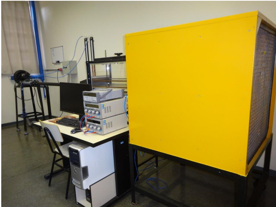
Túnel Aerodinâmico do Tipo Sucção de Retorno Aberto
