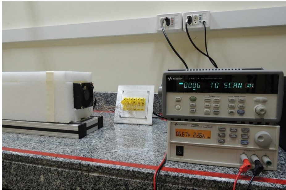
Resfriamento por convecção forçada em canal retangular horizontal
