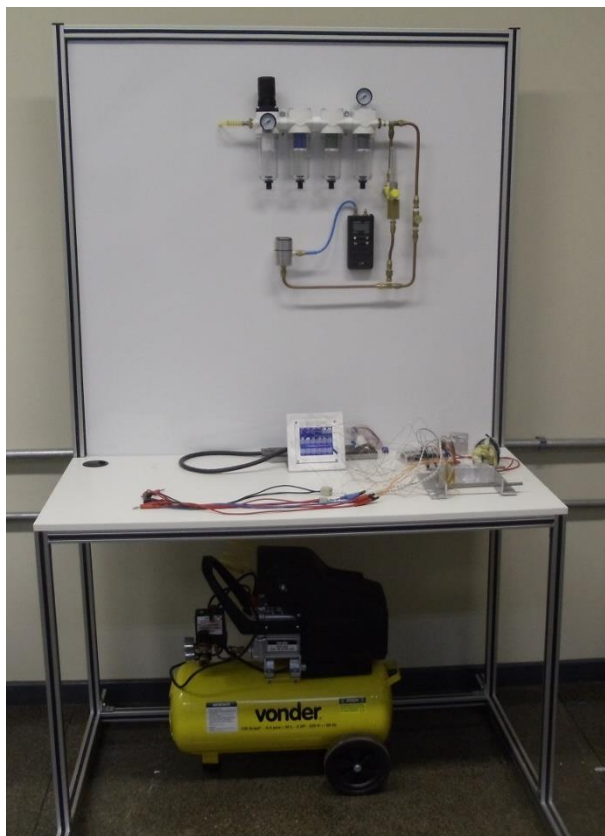
Bancada Experimental para Determinação de Permeabilidade, Porosidade, Raio Crítico e Condutividade Térmica
