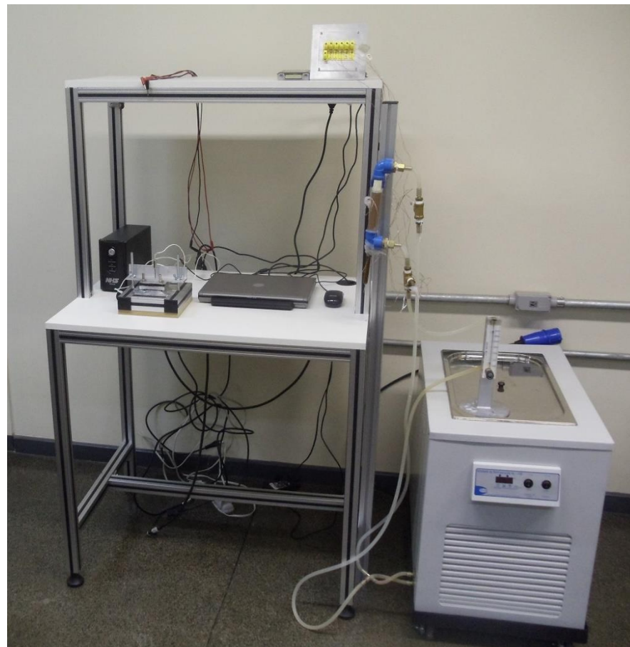
Desempenho Térmico de Termogeradores
