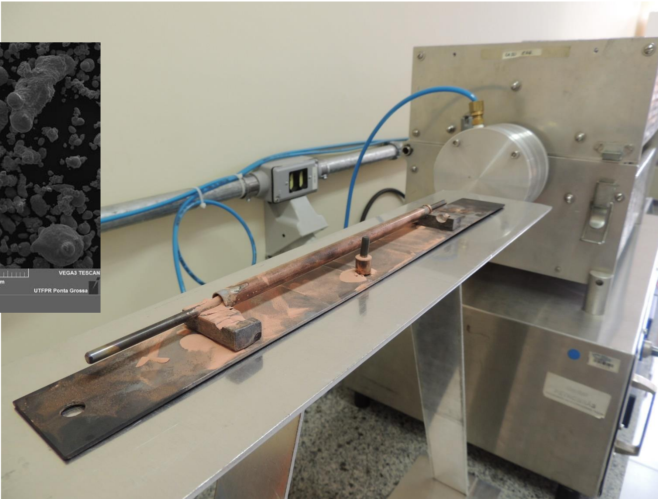
Sinterização de pó de cobre
